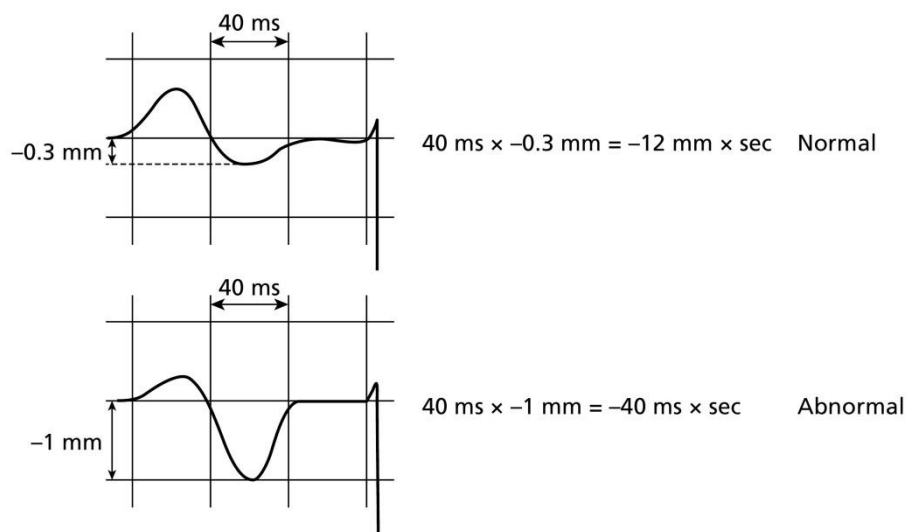
Hình 5.3: sơ đồ đối chiếu phần âm bình thường và bất thường của sóng P trong ở V1. Giá trị tính bằng chiều rộng (giây) và chiều sâu (mm) của phần âm vượt quá 40 ms x (-) mm thì được coi là bất thường.
