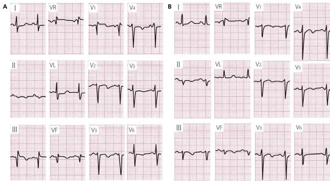
Hình 15.4: (A) một BN 59 tuổi với thuyên tắc phổi và hình thái McGinn – White điển hình: S_1 Q_{III} T_{III} âm. (B) các ECG sau khi BN hồi phục.
